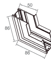
CONECTOR EN "L" VERTICAL EMPOTRADA PARA RIEL MÁGNÉTICA TIPO PERFIL Ref.: T2208L
