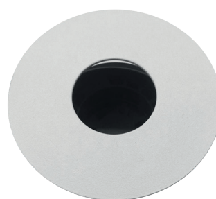
OJO DE BUEY PINHOLE EN "O" FIJO GU10 REDONDO / PLANO ALUMINIO Diámetro: Ø88mm Profundidad: 75mm Ref.: 2012-O
