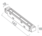
CONECTOR PARA RIEL MÁGNÉTICA Ref.: T22A03
