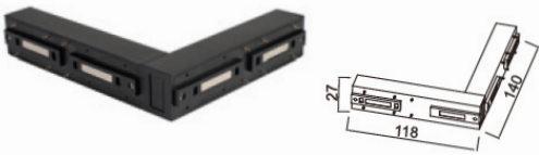
CONECTOR EN "L" EMPOTRABLE ÁNGULO INTERNO PARA RIEL MAGNÉTICA Ref.: T23L04
