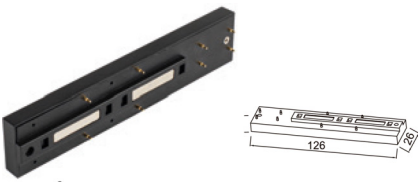
CONECTOR EN "L" HORIZONTAL PARA RIEL MAGNÉTICA ULTRADELGADA Ref.: T23A03
