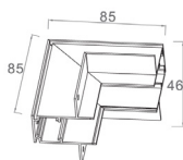
CONECTOR EN "L" VERTICAL EMPOTRADA PARA RIEL MÁGNÉTICA Ref.: T2206L
