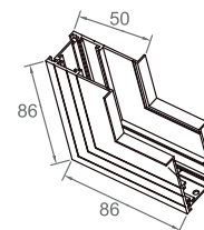
CONECTOR EN L 90° EMPOTRABLE PARA RIEL MAGNÉTICA TIPO PERFIL Ref.: T2208L Cod.: 010972
