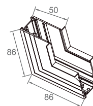
CONECTOR EN L 90° EMPOTRABLE PARA RIEL MAGNÉTICA TIPO PERFIL Ref.: T2208L Cod.: 010972
