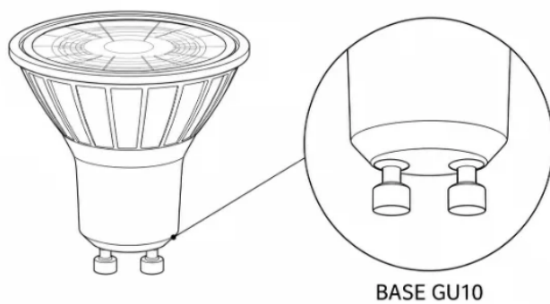
Diagrama · Identificación de base GU10 (dos terminales)
