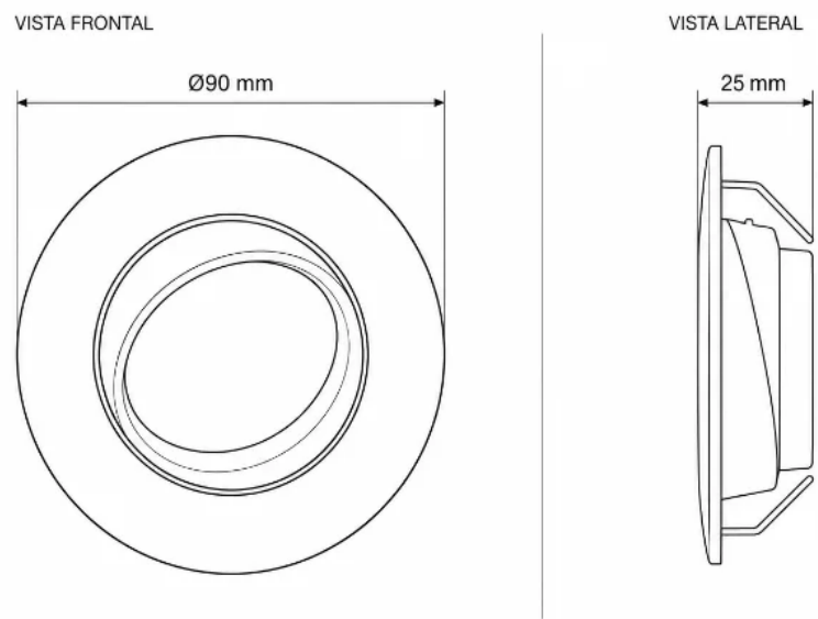
Diagrama · Dimensiones (vista frontal Ø90 mm · vista lateral 25 mm)
